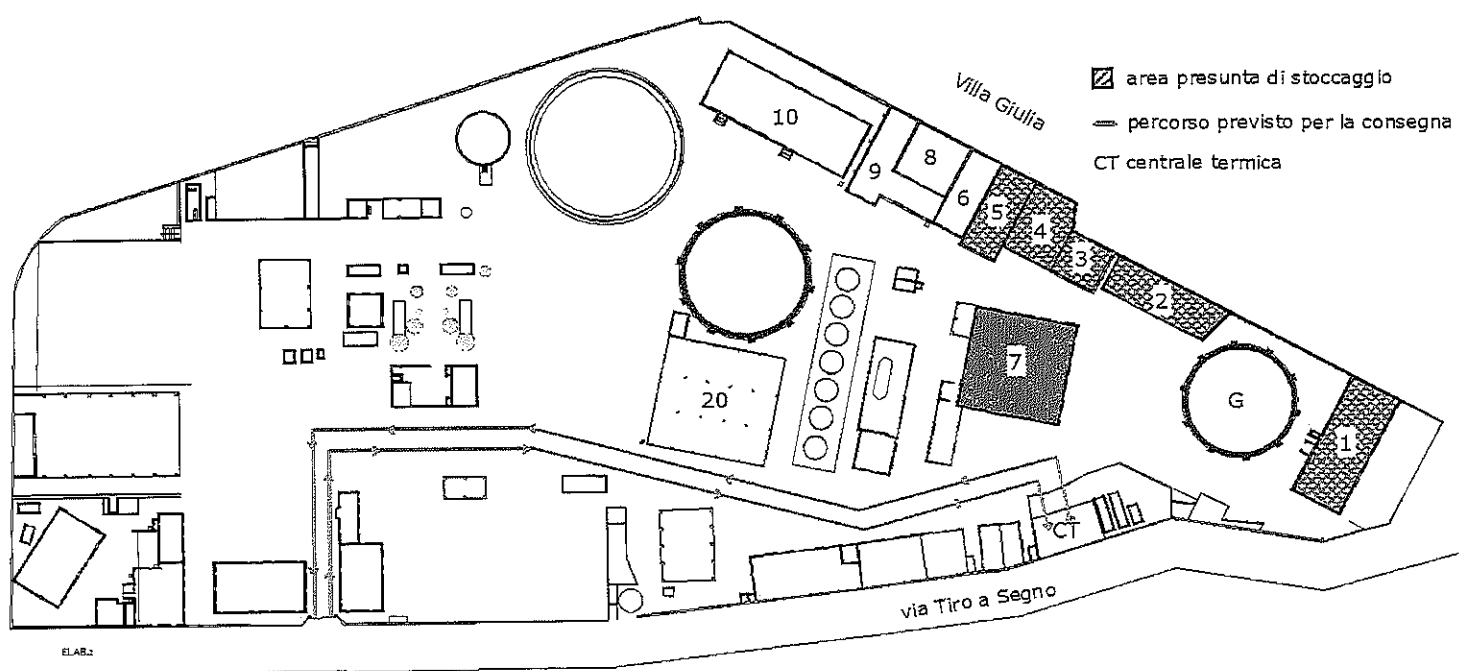
Area di consegna ed installazione delle apparecchiature e percorso previsto
