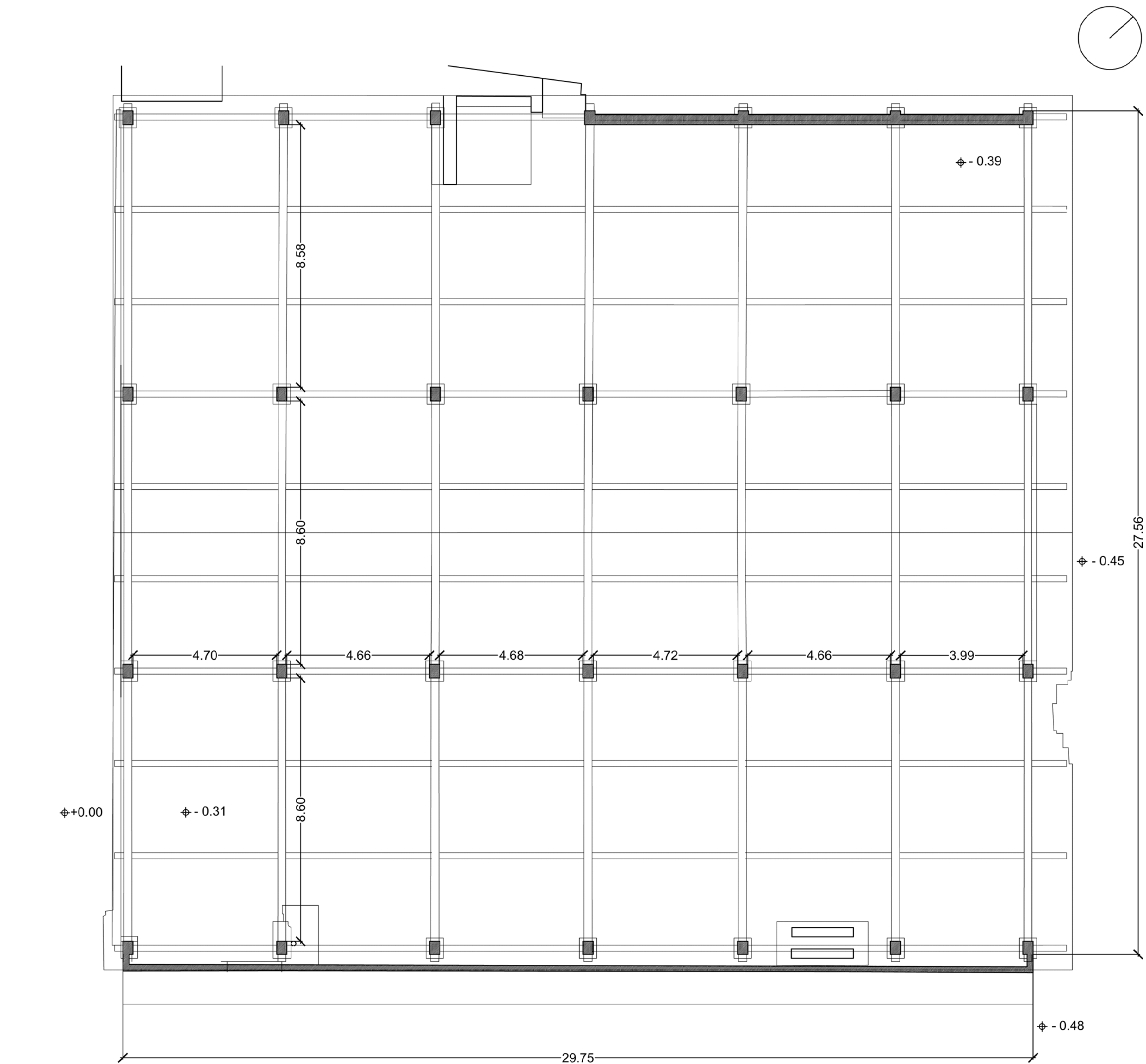
Pianta
