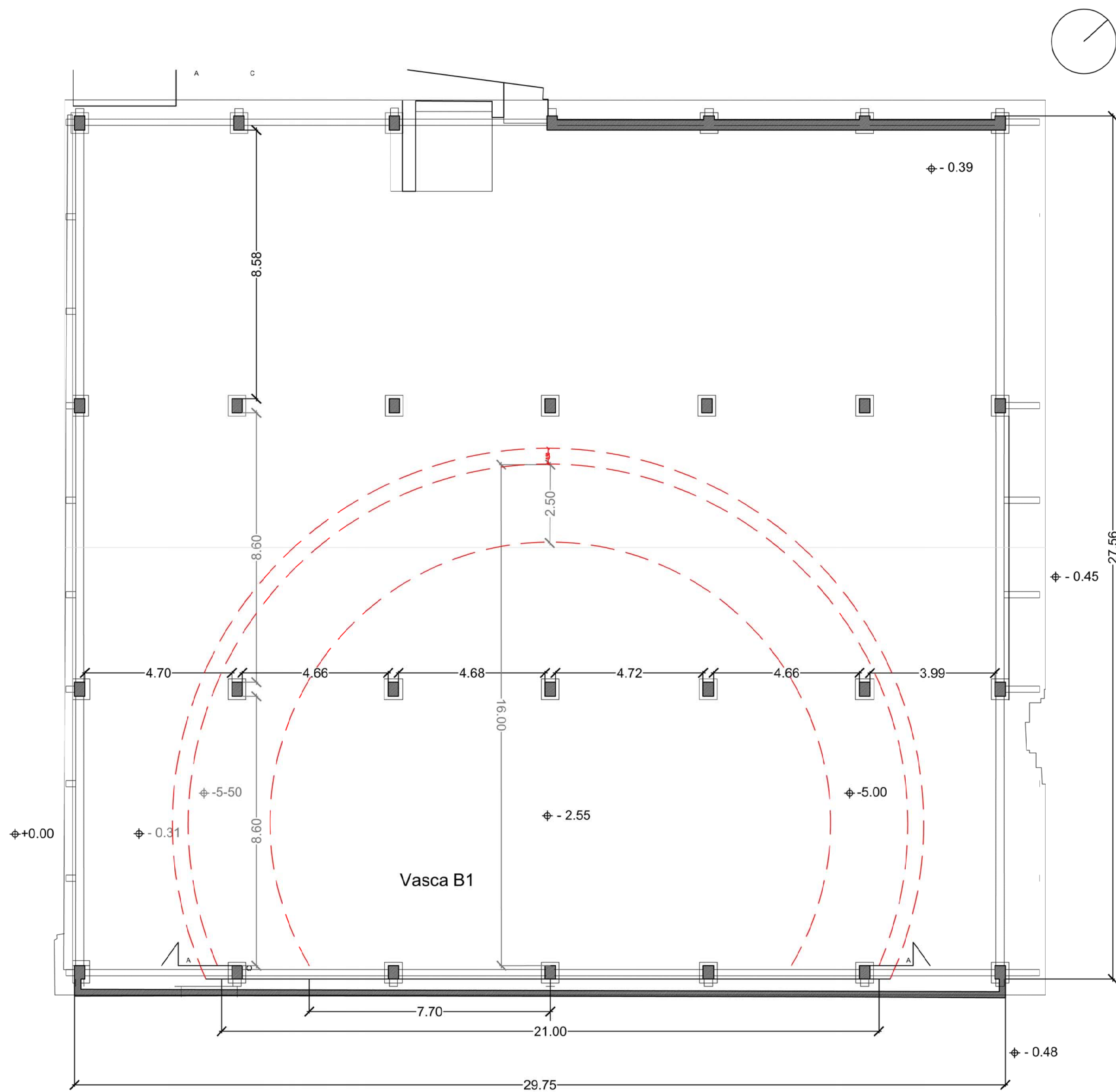
Pianta
