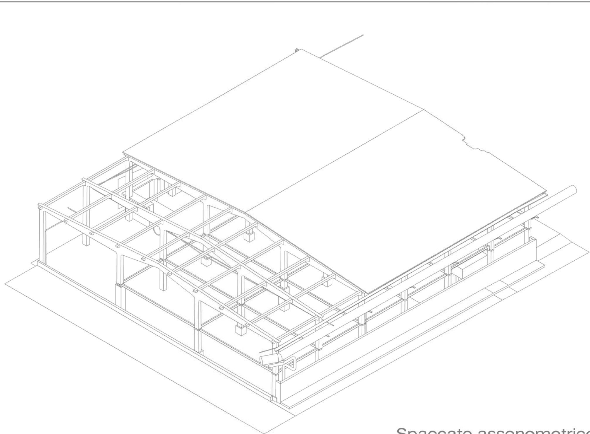
Spaccato assonometrico
