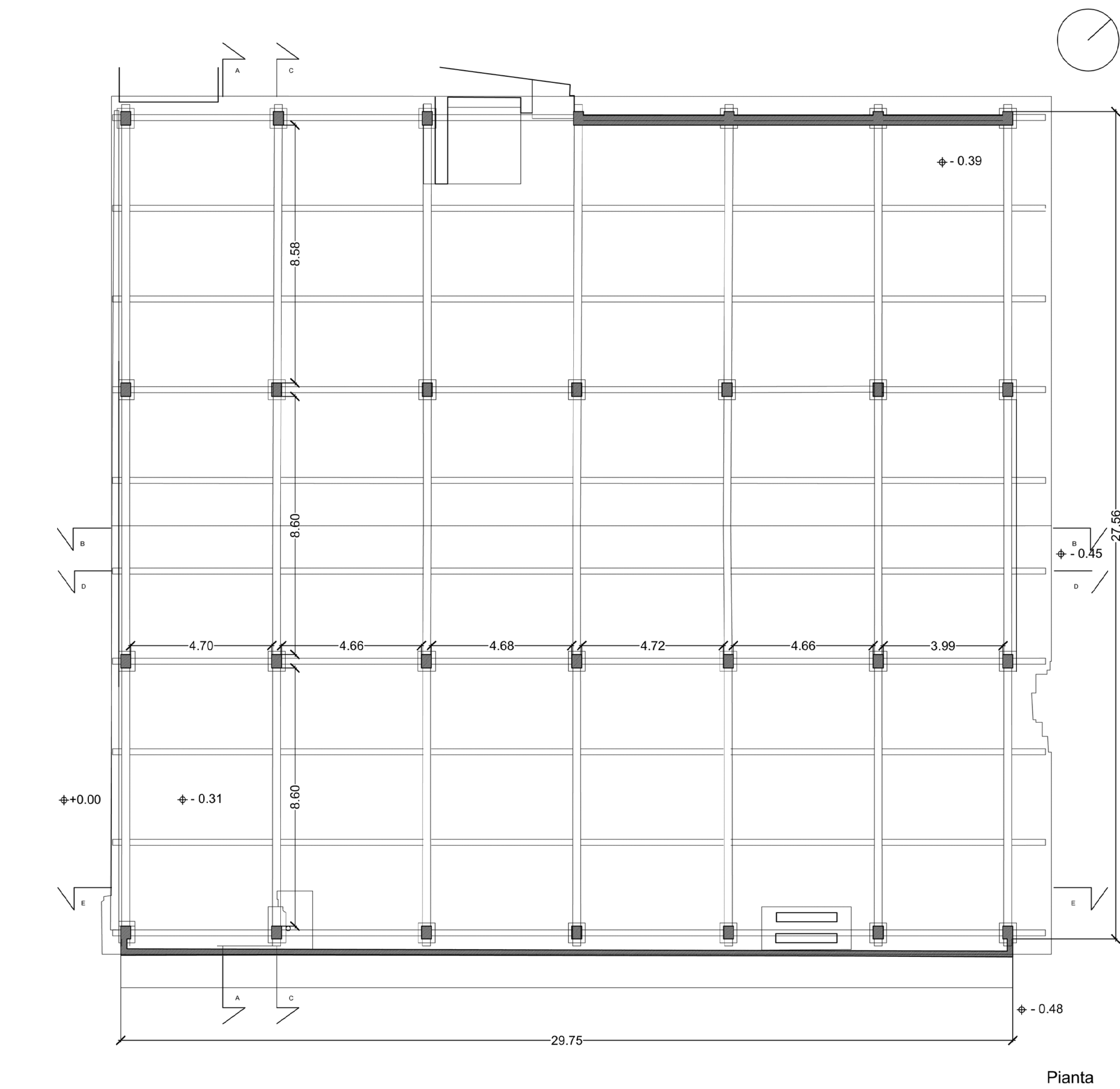
Pianta
